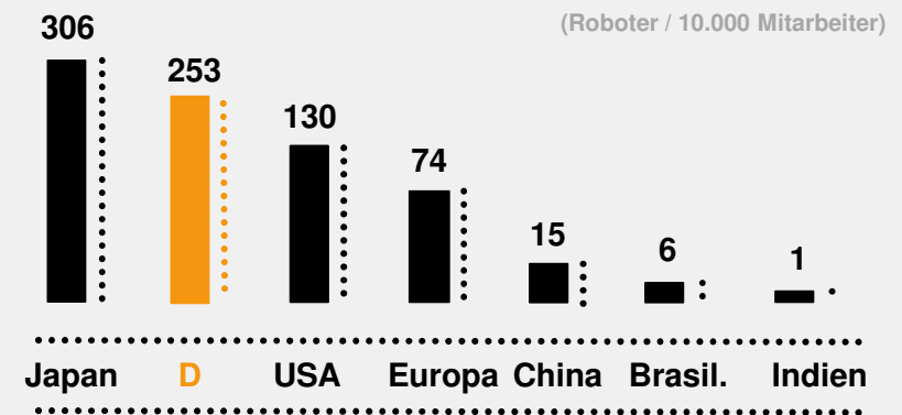
Roboterdichte (IFR 1 )
